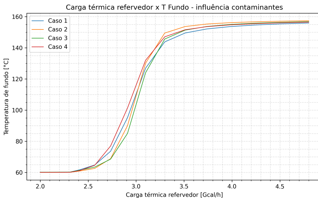
Figura 3: Carga térmica x temperatura do fundo - Influência Contaminantes
