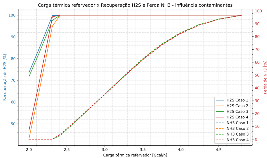
Figura 1: Carga térmica x recuperação de \text{H}_2\text{S} e perda de \text{NH}_3
